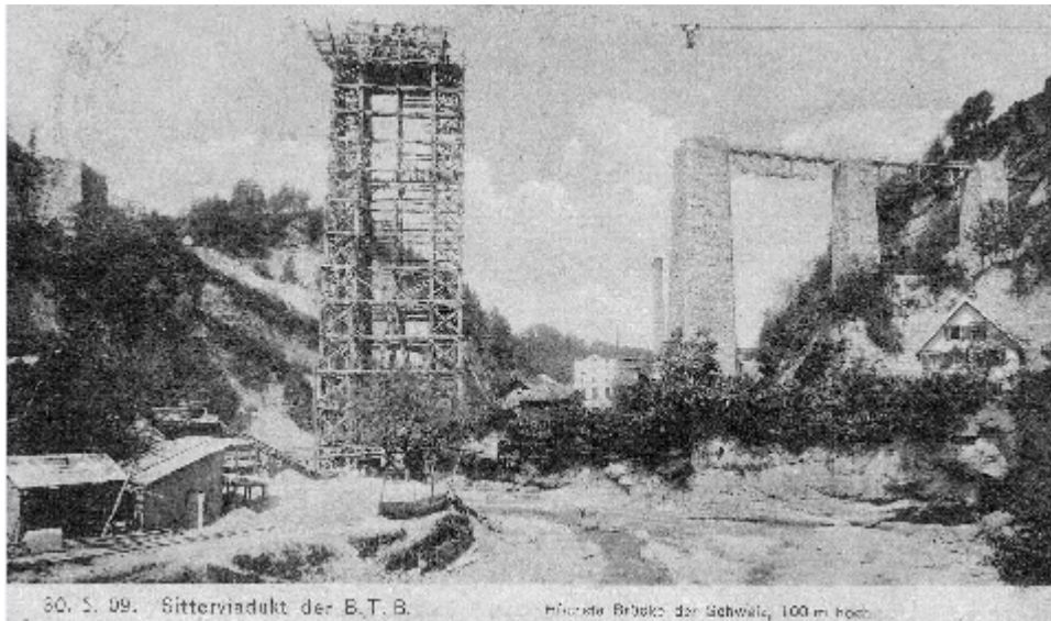
Bau des Sitter-Viaduktes der Bodensee-Toggenburg-Bahn, St. Gallen, 30.5.1909
